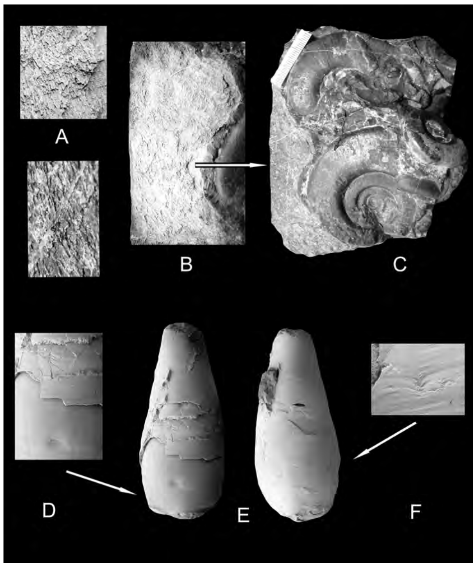
Tabule 1. Kusy byly před fotografováním poběleny chloridem amonným. Měřitko zobrazuje 20 mm. Table 1. Fossils were coated with ammonium chloride before photographing, scale bar represents 20 mm.
